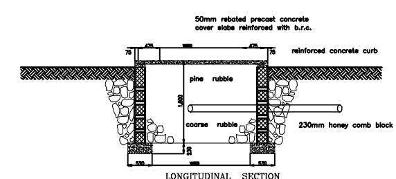
LONGITUDINAL SECTION
