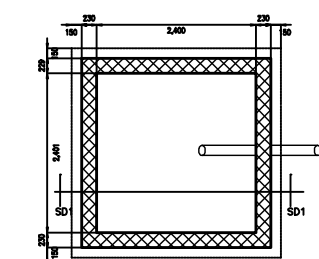
SOAKAWAY (PLAN)
